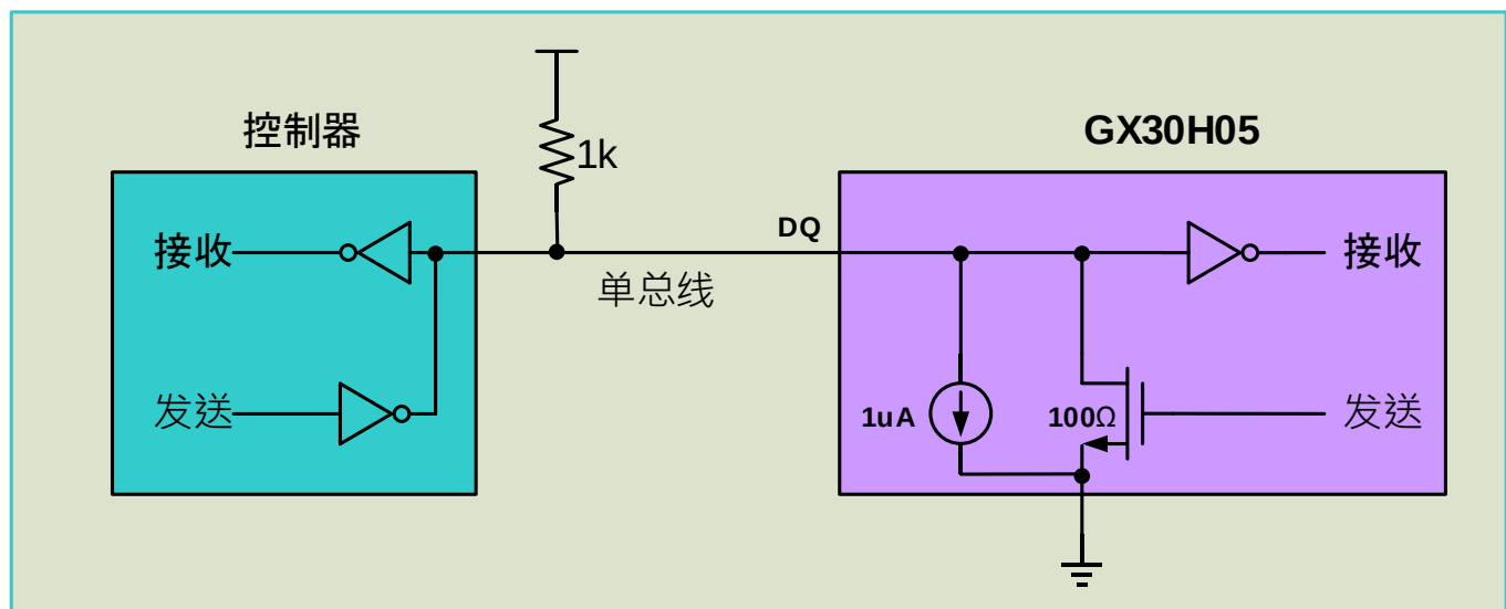
图 10. 硬件结构图
