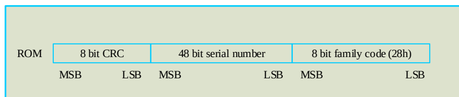
图 6. 64 位 ROM 码
