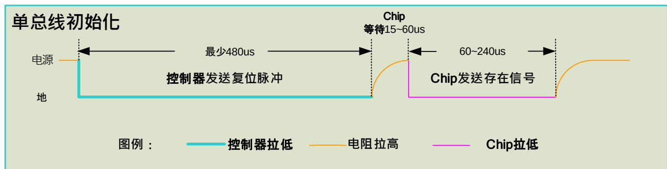
图 13. 初始化序列
