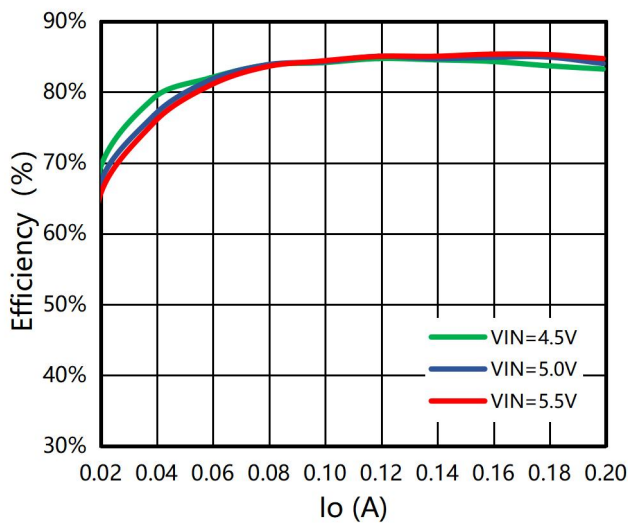
效率 VS 输出电流(输出满载@105°C)
