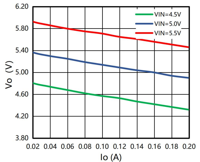
输出电压 VS 输出电流(105°C)
