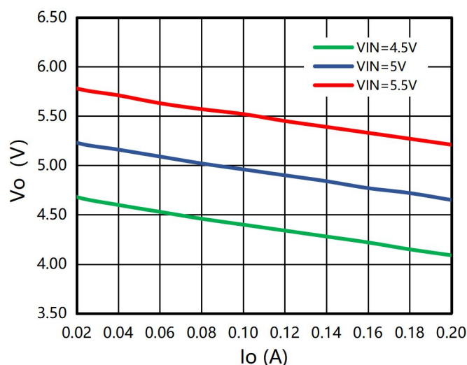
图 3: 输出电压 VS 输出电流
