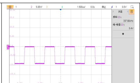
VIN=4.5V, 满载工作电压波形
