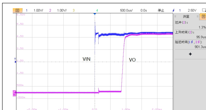
图 4: VIN=5V, 满载启机波形
