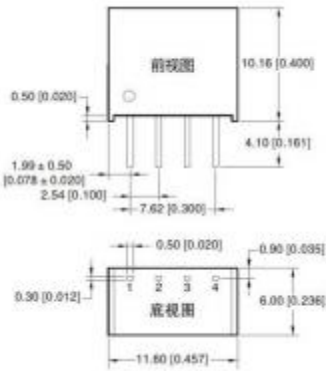
图4：外型尺寸
